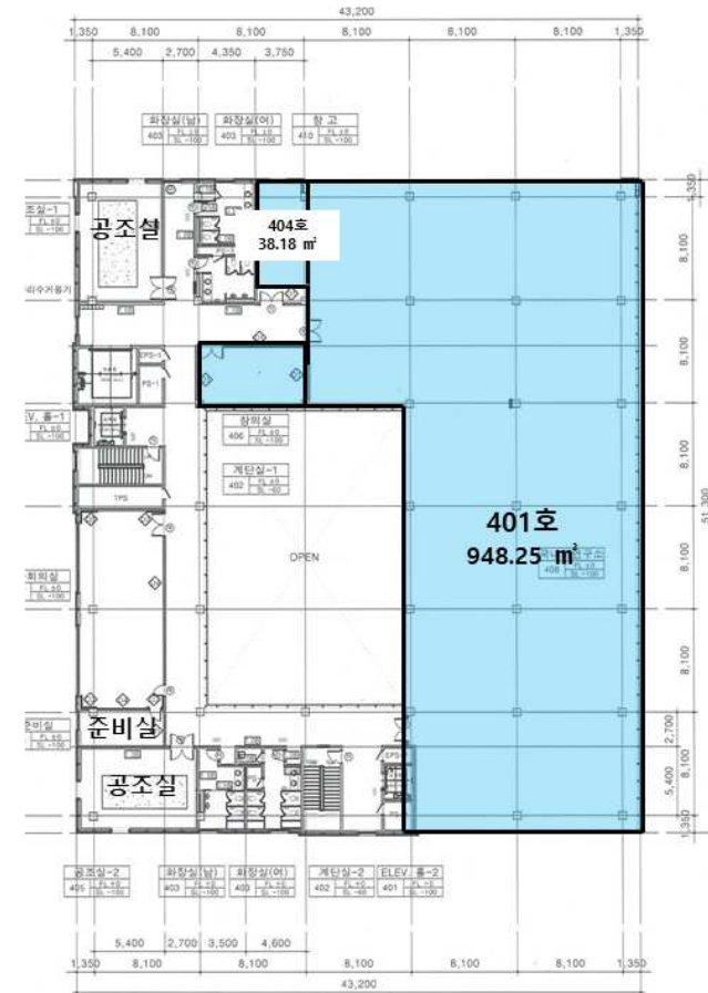
2 지상4층 평면도 SCALE: A1: 1/200 A3: 1/400
