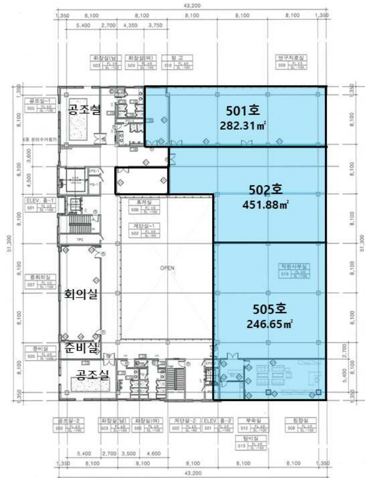
1 지상5층 평면도 SCALE : A1 : 1/200 A3 : 1/400
