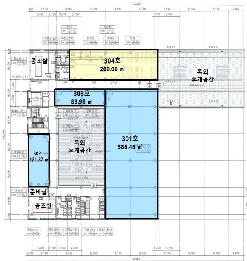
1 지상3층 평면도 SCALE: A1: 1/200 A3: 1/400
